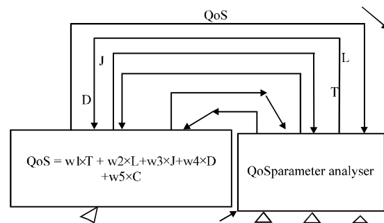
Fig. 5: QoS parameter analyzer
