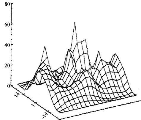
Fig. 6: A 3D of \beta_0 values versus longituede and latitude
